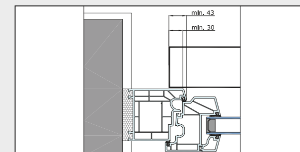
Platzbedarf seitlich
