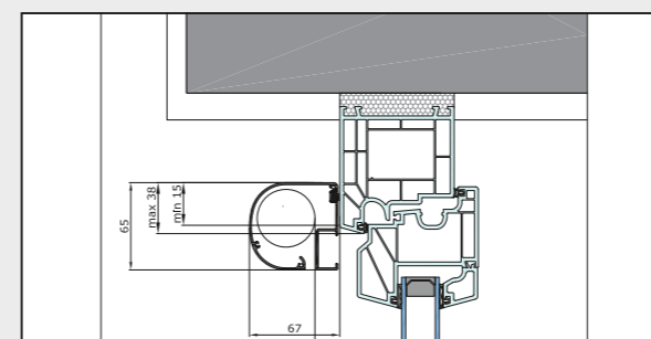
Platzbedarf oben
