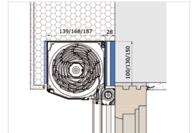
Mit Wärmedämmverbundsystem und Sturzdämmung VORO WDVS mit integriertem IGI-Rollo
