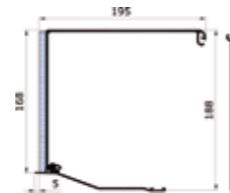
Größe 18 Rollladen | Raffstore 80R
